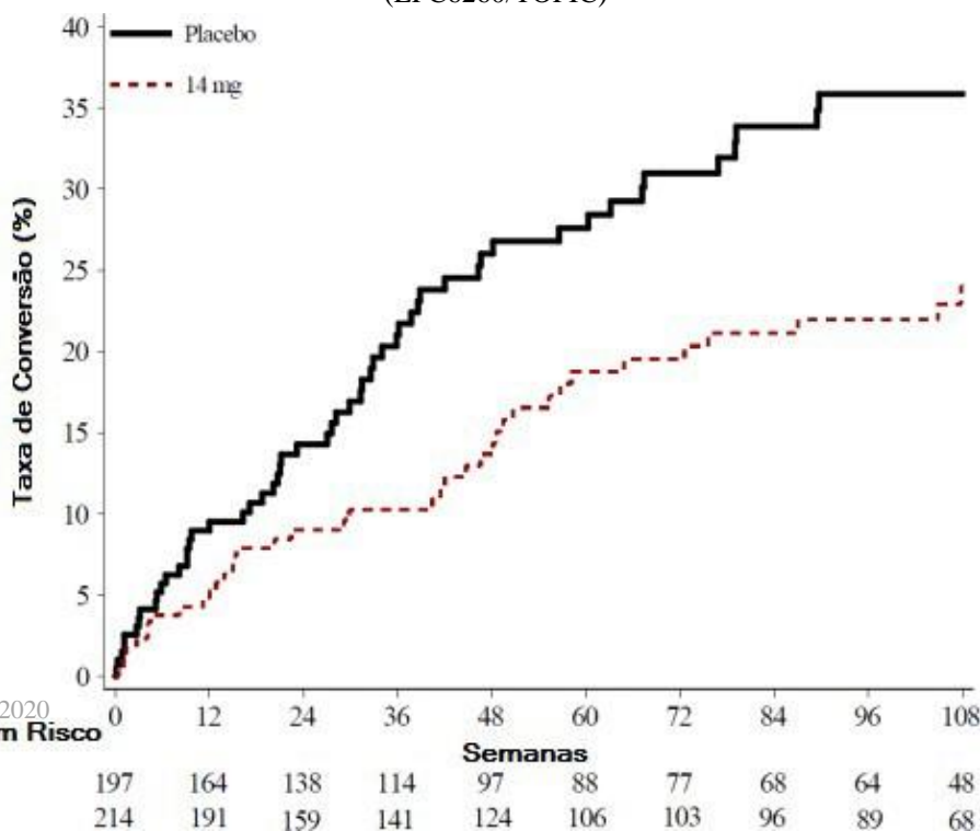
Figura 3: Gráfico Kaplan-Meier do tempo para o segundo episódio clínico – população com intenção de tratar (EFC6260/TOPIC)
